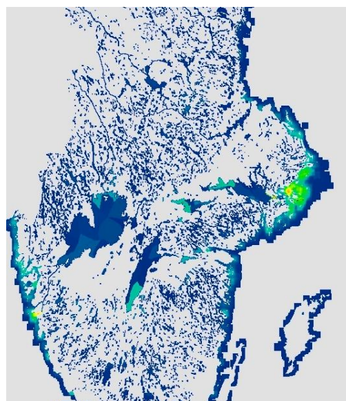
Figur 12. Fördelningen av emissioner från småbåtar. Gul och grön färg markerar höga emissioner och blå färg låga emissioner.
