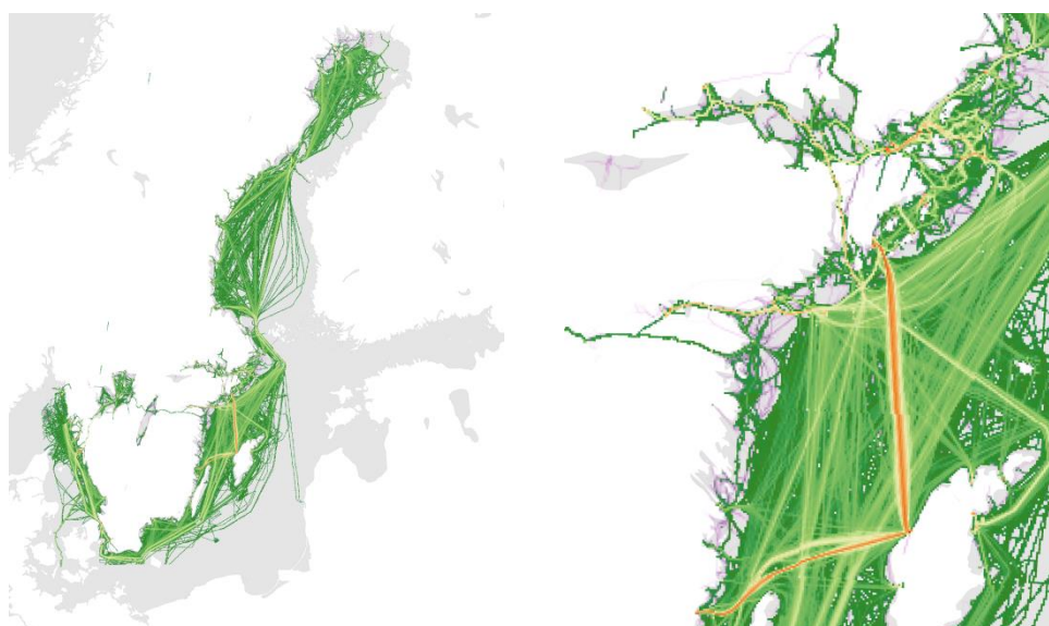
Figur 9. Fördelning av NO x -emissioner ifrån inrikes sjöfart i Östersjön och Västerhavet (vänster) och en förstoring över Stockholm och Gotland (höger). Röd färg markerar höga emissioner och grön färg låga emissioner.
