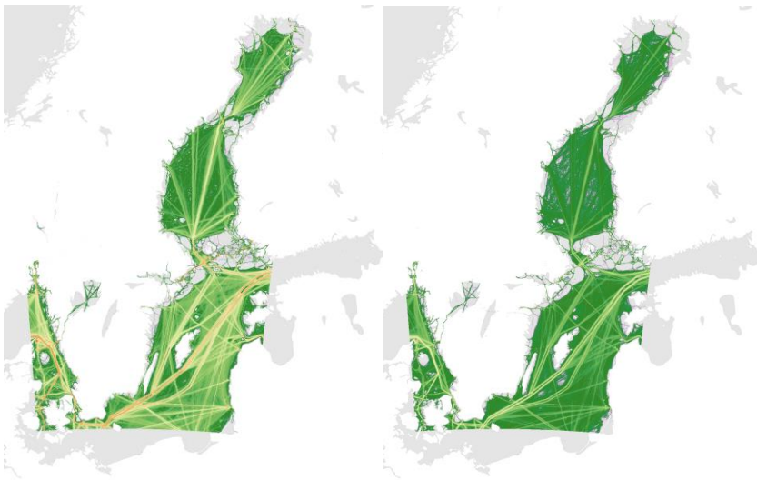
Figur 24. Fördelning av SO x -emissioner från internationell sjöfart i Östersjön och Västerhavet för åren 2014 (före skärpta svavelregler) och 2015 (efter skärpta svavelregler). Röd färg markerar höga emissioner och grön färg låga emissioner.
