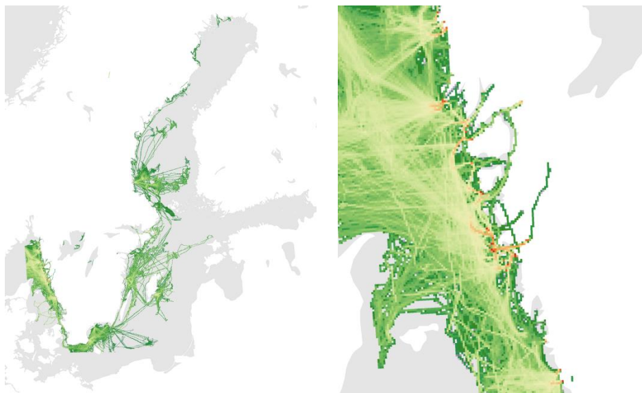
Figur 17. Fördelningen av utsläpp av CO 2 från fiskefartyg i inrikes trafik i Östersjön och Västerhavet (vänster) och i Skagerrak (höger). Röd färg markerar höga emissioner och grön färg låga emissioner.
