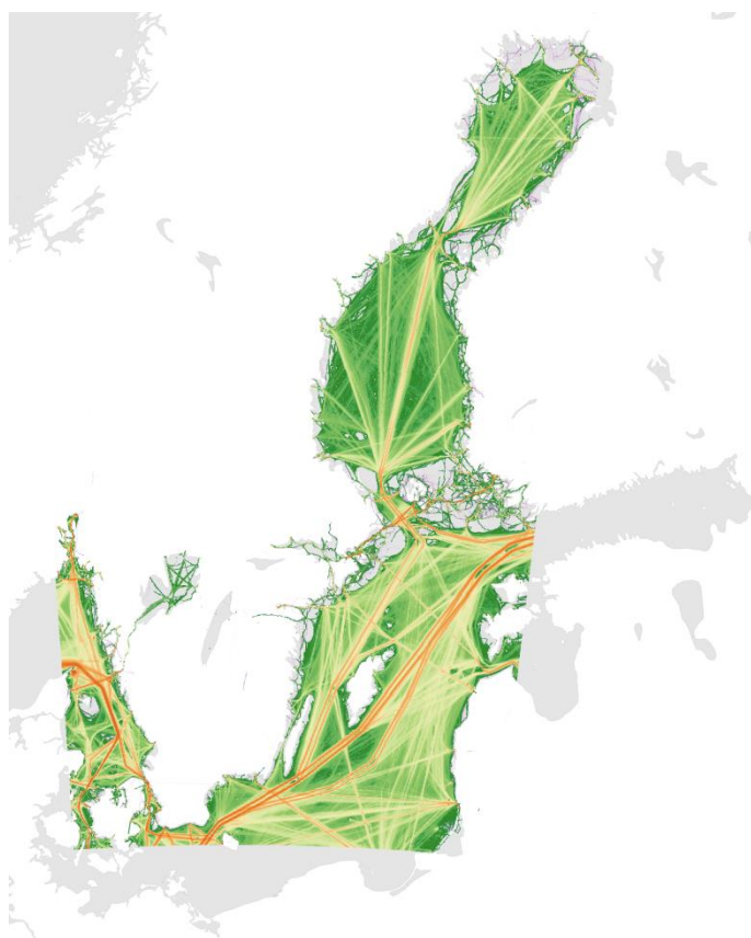
Figur 25. Fördelning av NO x -emissioner från internationell sjöfart i Östersjön och Västerhavet under 2016. Röd färg markerar höga emissioner och grön färg låga emissioner.
