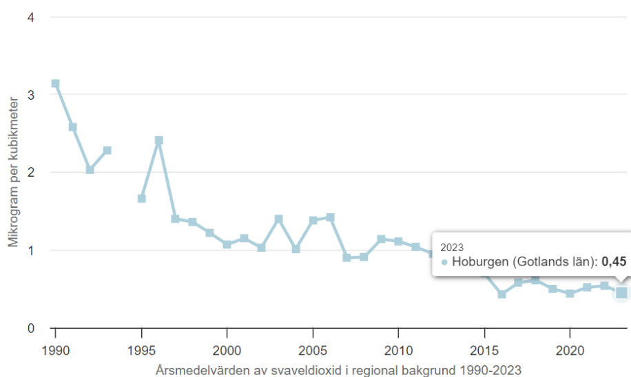
Bild 1: Diagrammet visar den minskade trenden av svavelhalt i luften, från mätningar vid Hoburgen, Gotland. Källa: Naturvårdsverket.
